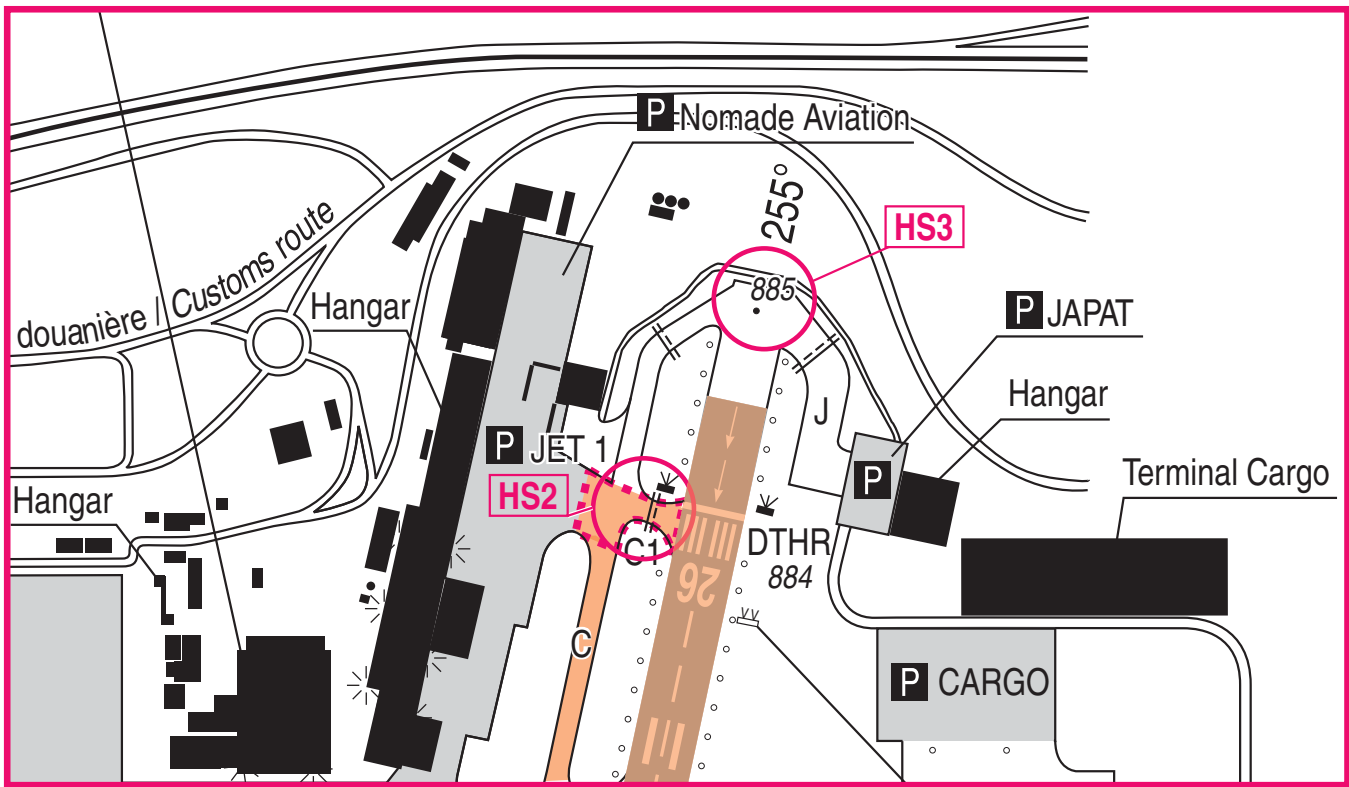
Extrait carte AD 2 LFSB ADC 01 en vigueur le 27 février 2020
