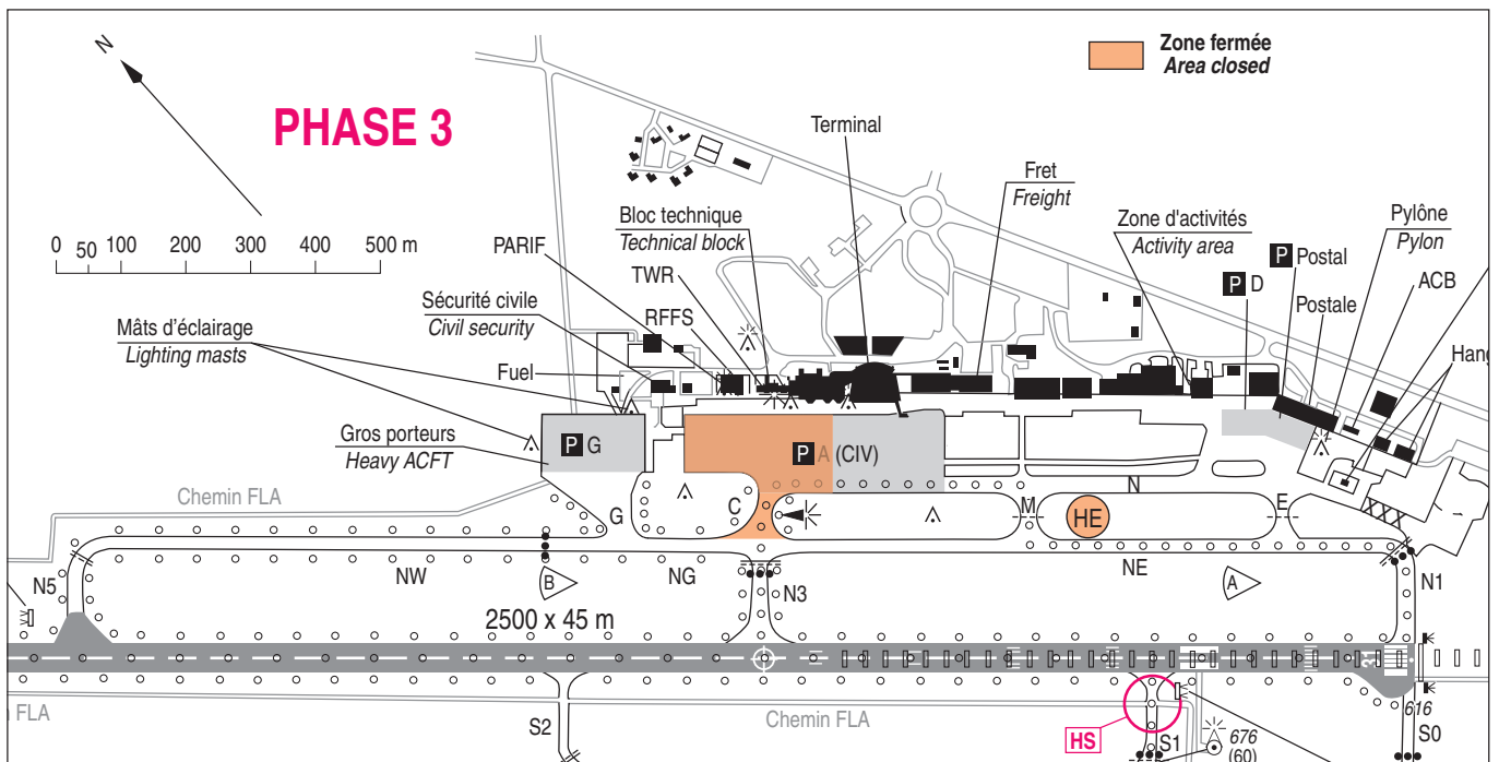
Excerpt from AIP France « AD 2 LFBP ADC 01 » WEF 18 JUN 2020
