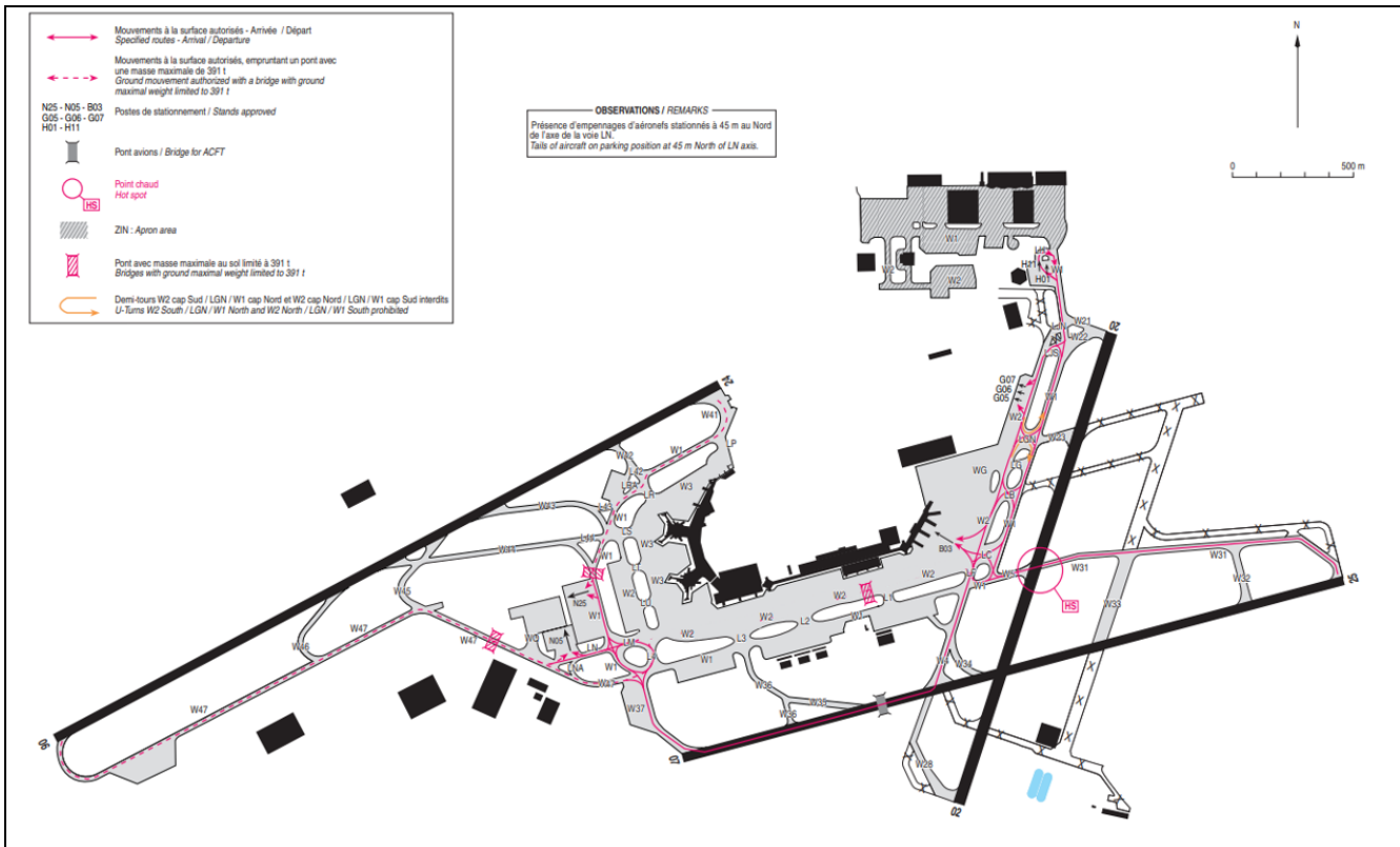
Extrait carte AD 2 LFPO GMC 04
