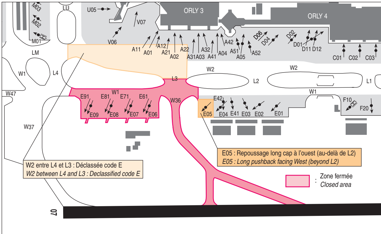
Extrait carte AD 2 LFPO APDC 01
