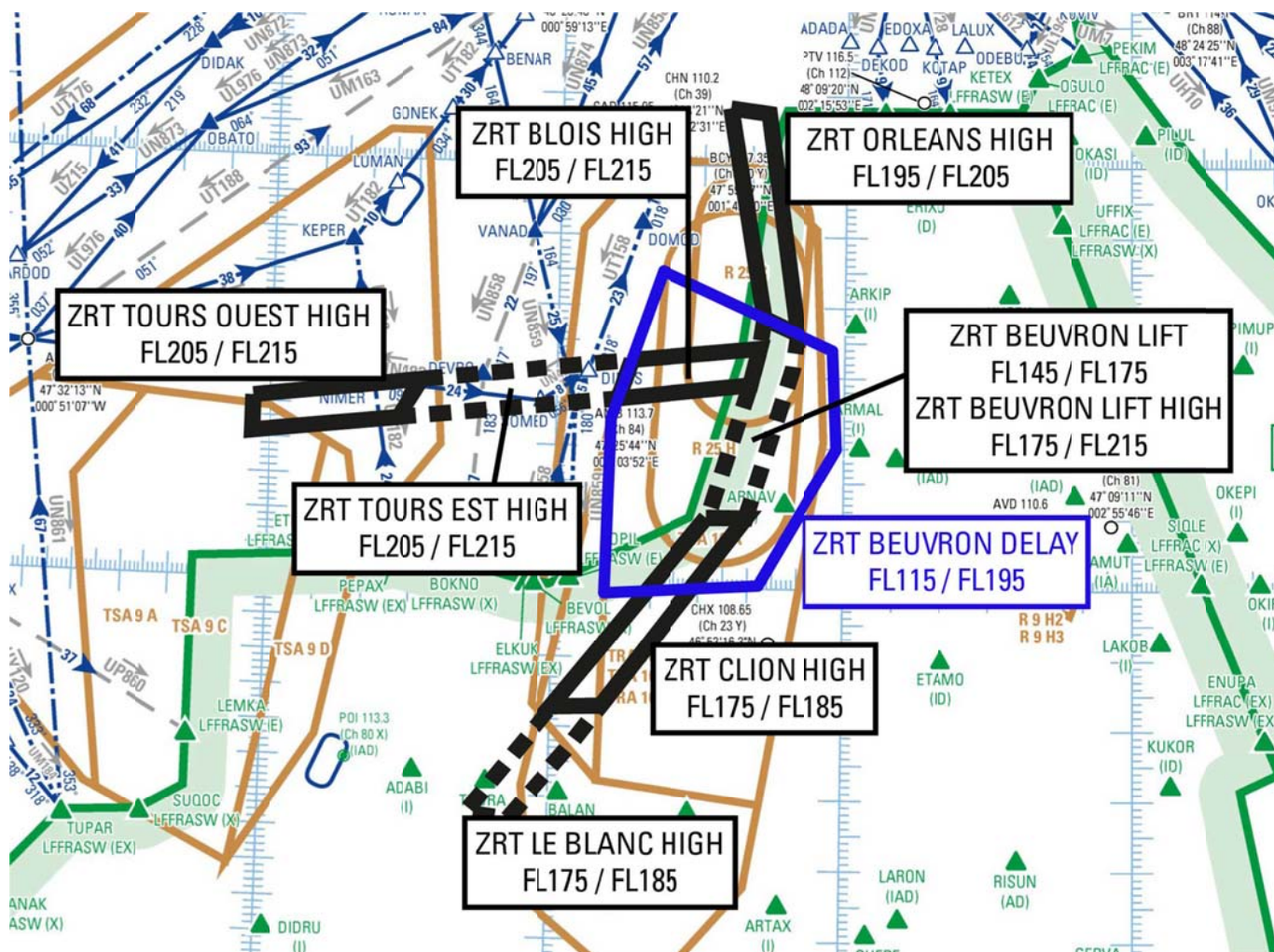
Extrait carte de croisière ENR 6.2 Édition 24/02/2022
