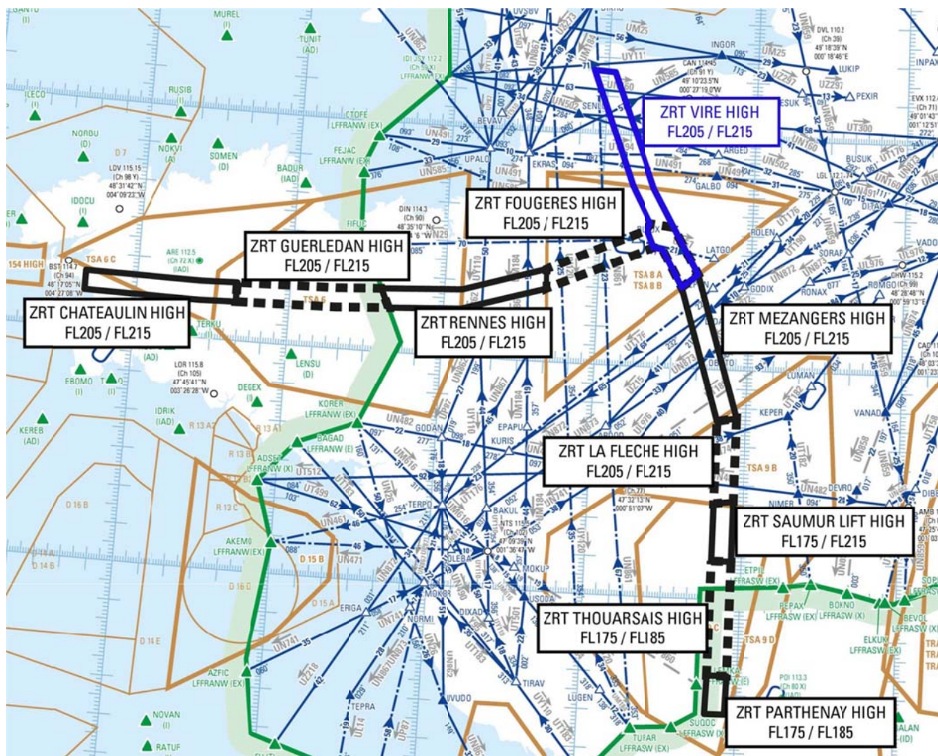
Extrait carte de croisière ENR 6.2 Édition 24/02/2022
