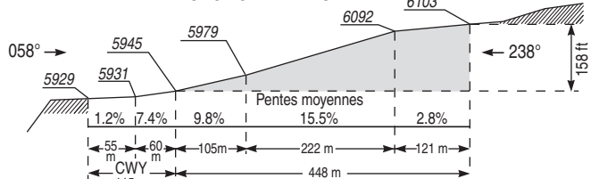
PROFIL EN LONG DE LA PISTE RWY LONGITUDINAL PROFILE
